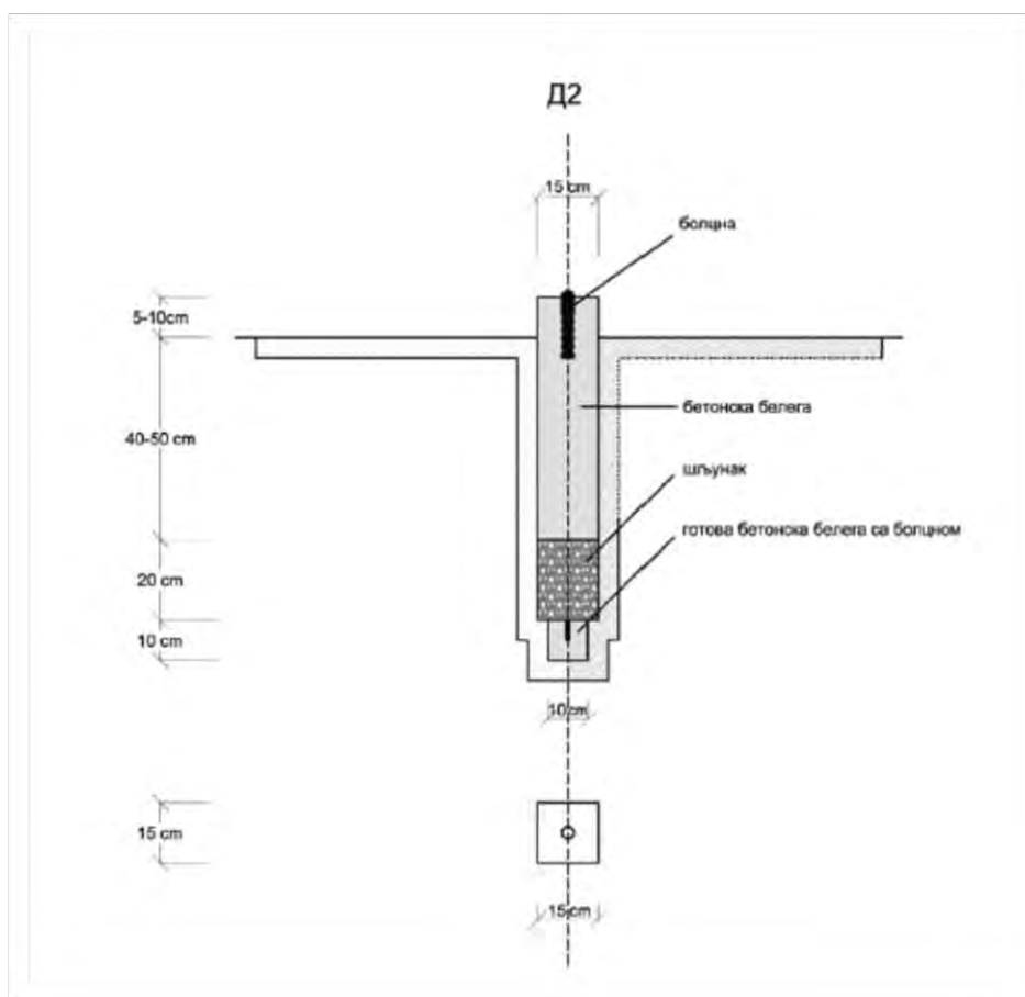
Слика 15: Изглед и димензије белеге ТИП Д2 са подземним центром
