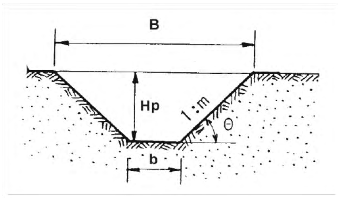
Слика 13: Изглед профила канала
