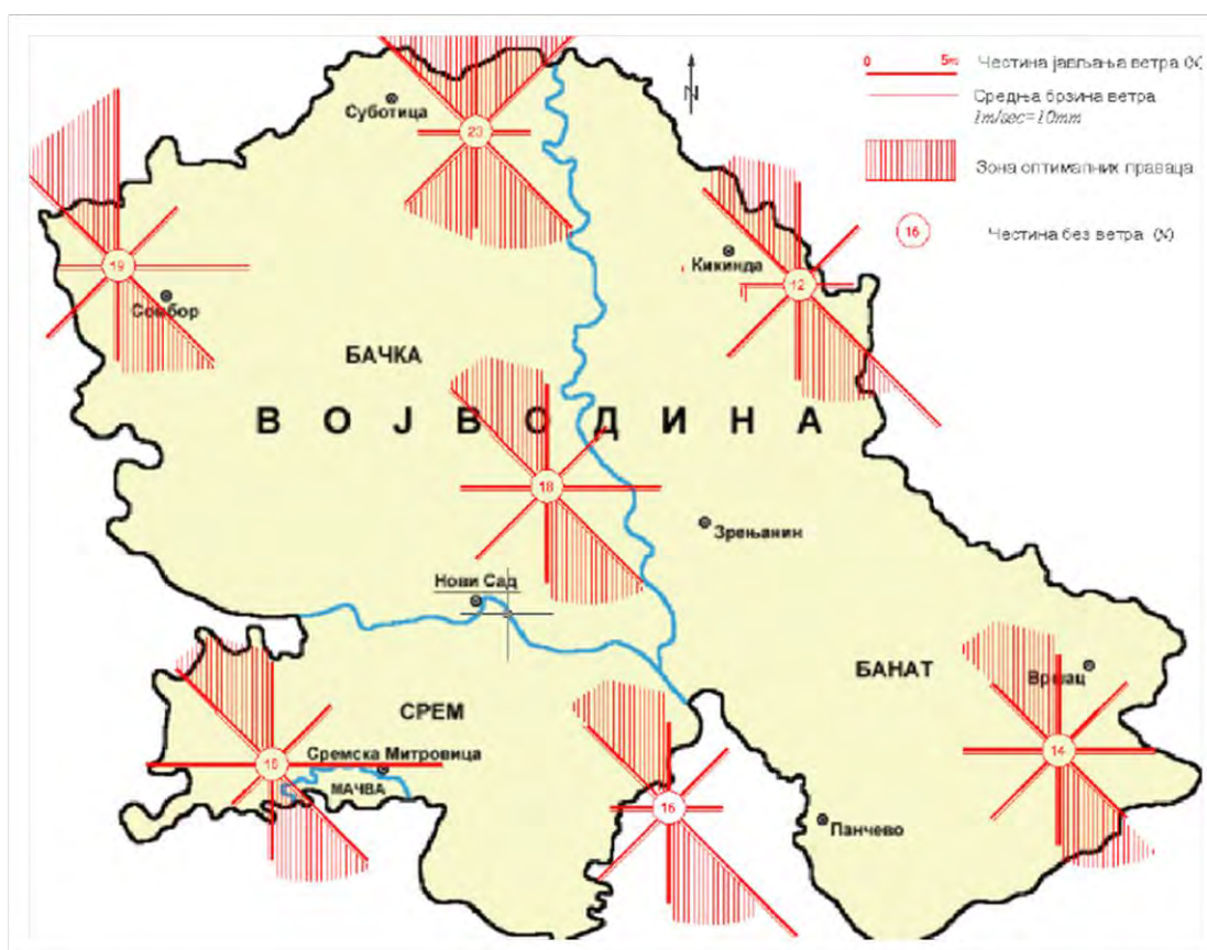
Слика 12: Оптимални правци дуже стране парцеле за подручје Војводине
