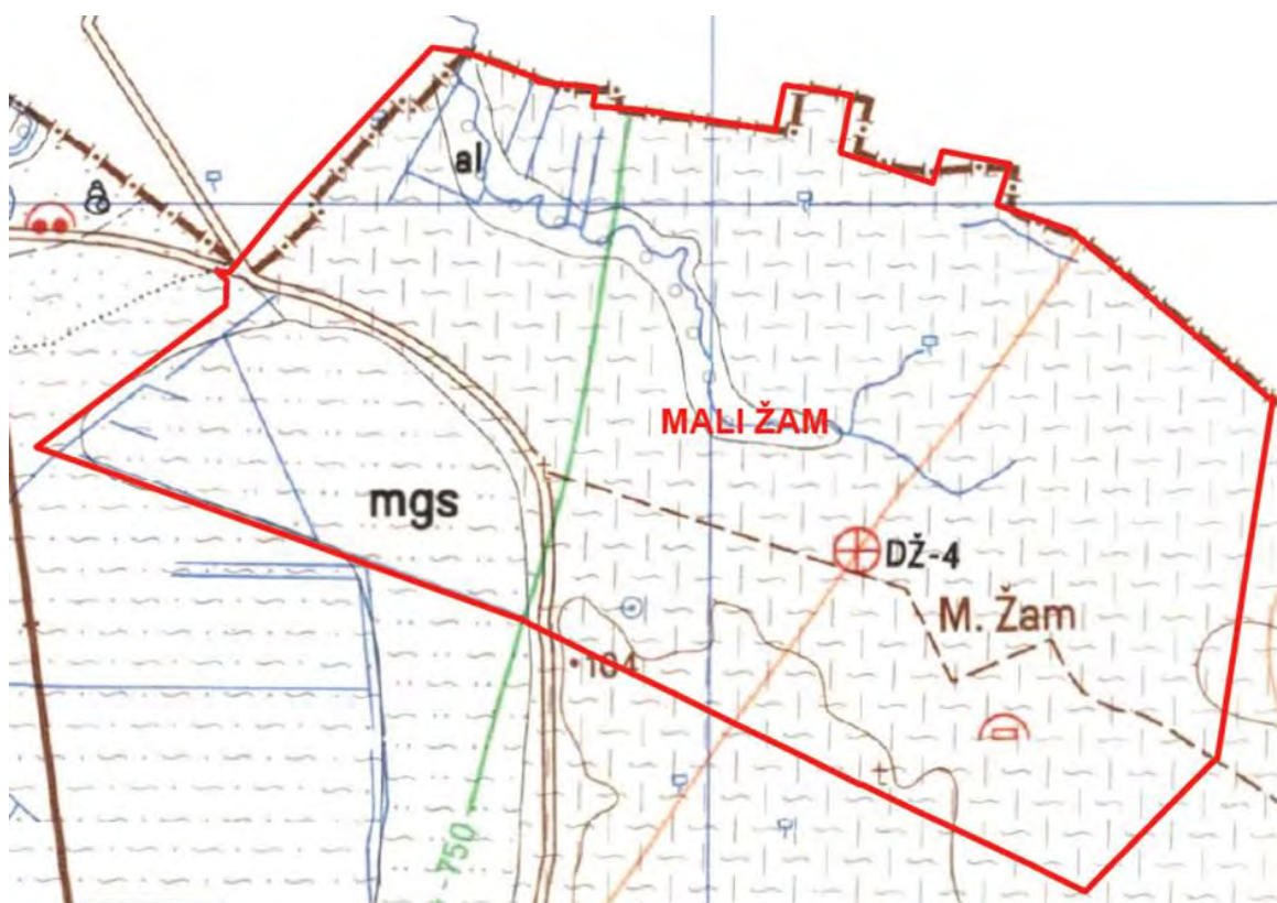
Слика 4: Геолошка карта КО Мали Жам
